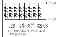
线路原理图
