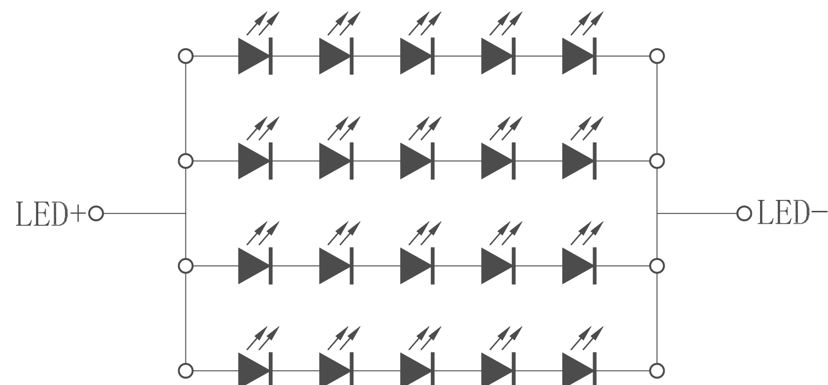
背光电路图 (CIRCUIT DIAGRAM)
