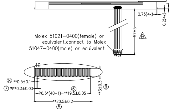
SECTION A 2:1
