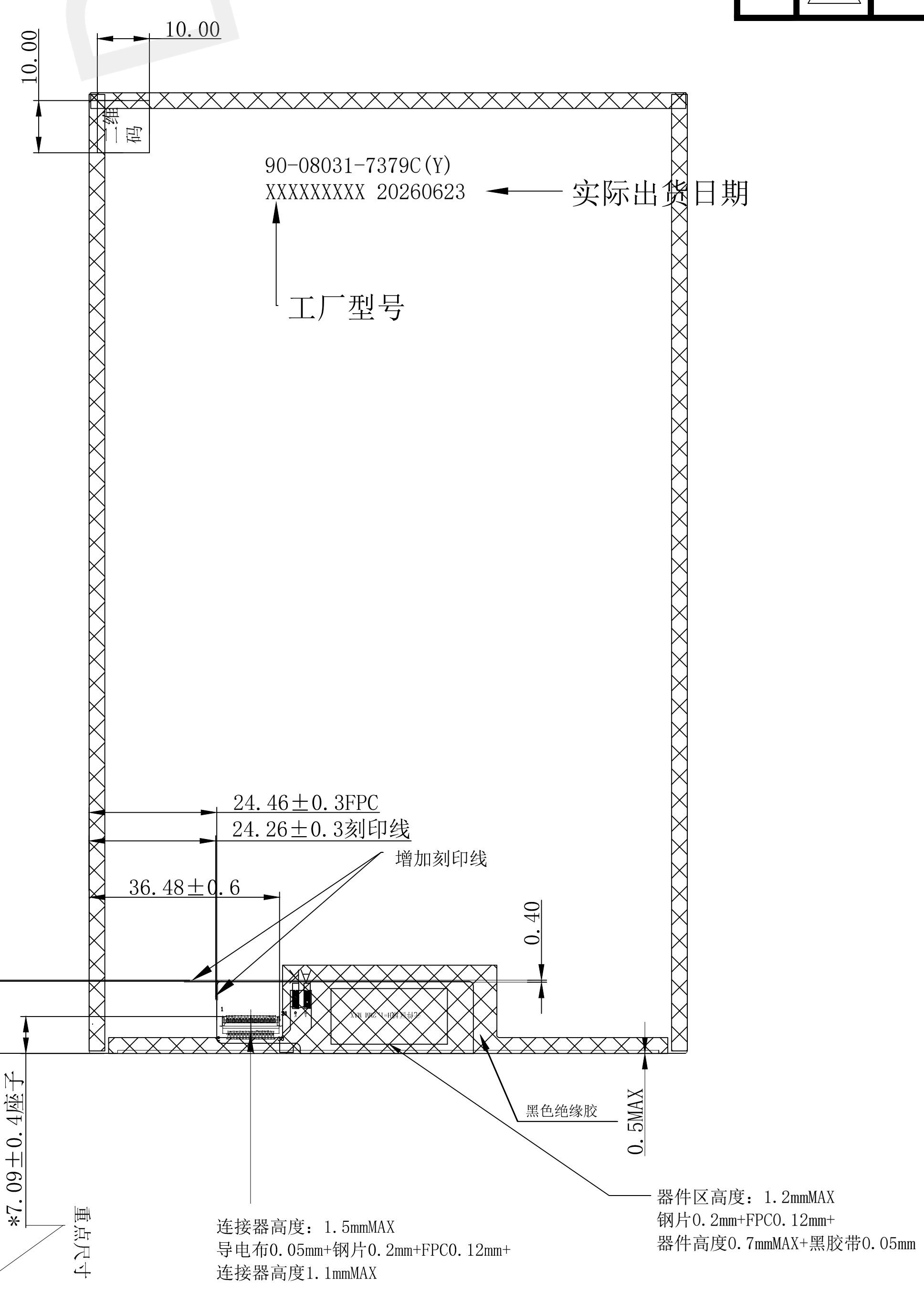
弯折示意图 排线弯折出货 连接器盖子闭合出货
