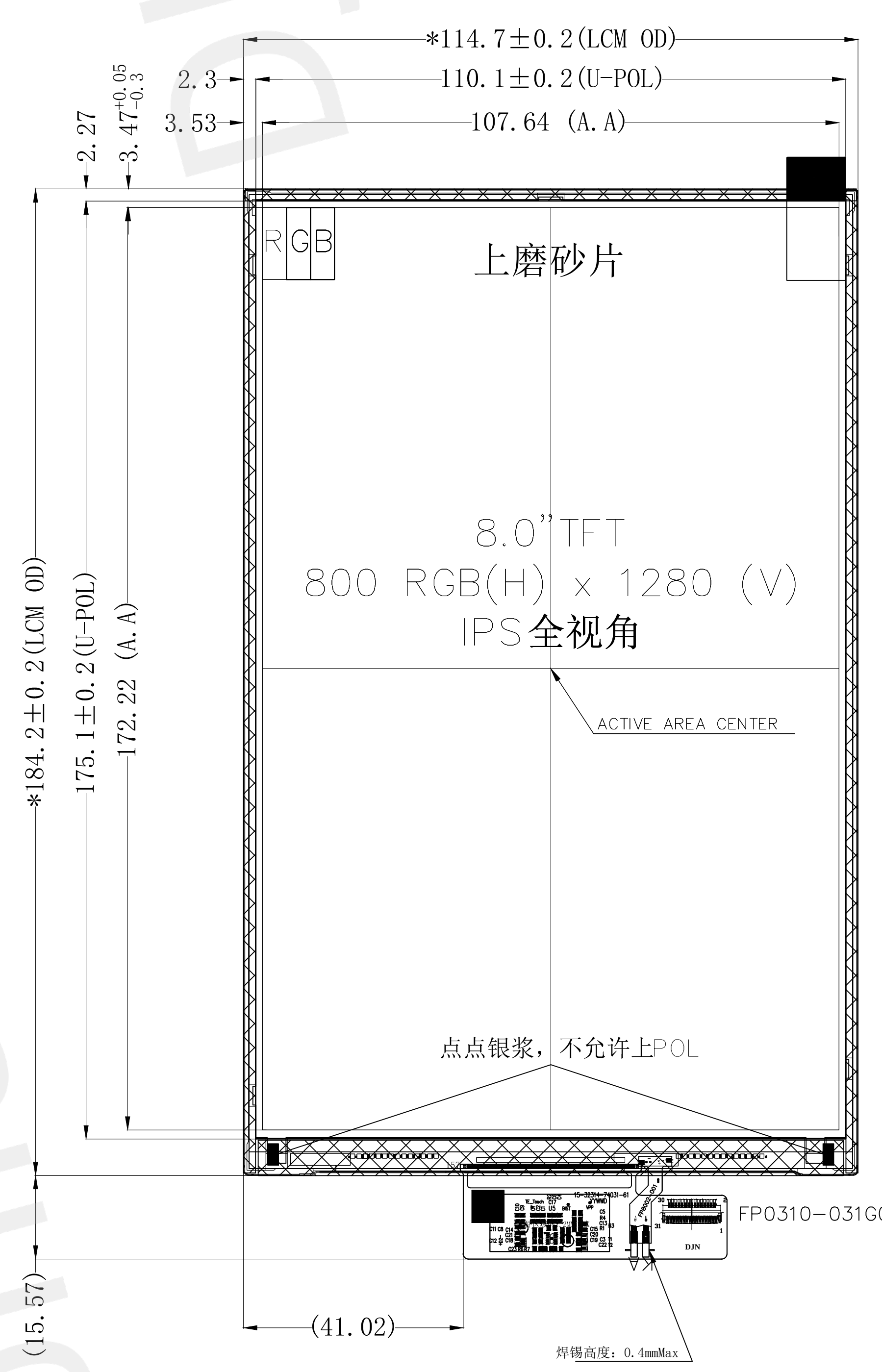
正视图
