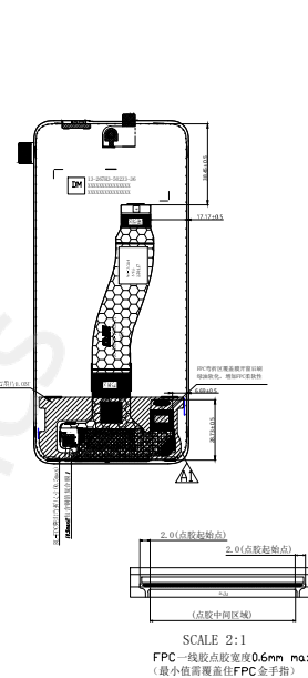
FPC弯折出货图
