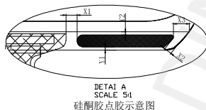
硅酮胶点胶示意图
