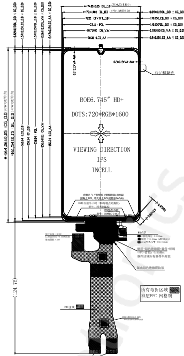
主视图
