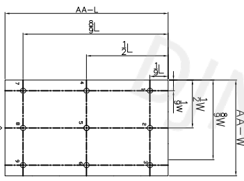
测试点分布9点(1/9)示意图
