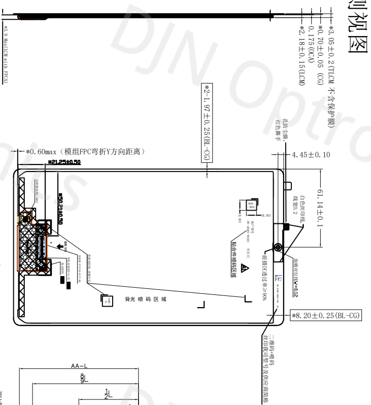
FPC弯折示意图 FPC弯折出货
