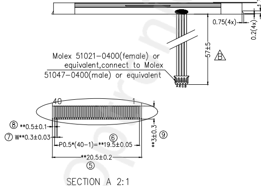
SECTION A 2:1
