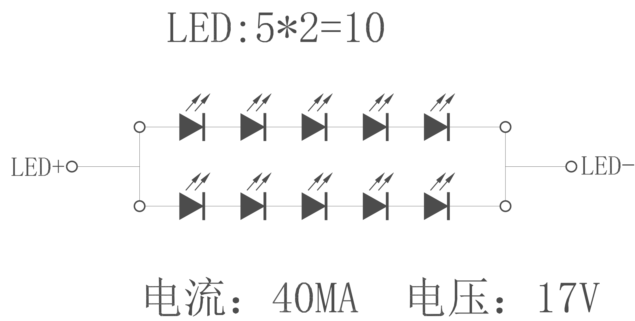
背光电路图 (CIRCUIT DIAGRAM)
